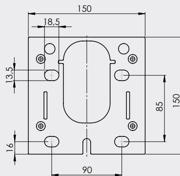
Golvplatta för stolpe
