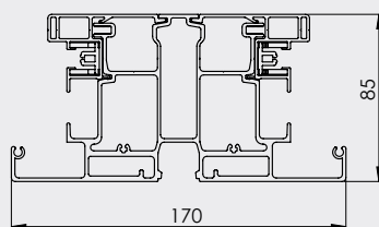
Dubbelskena
