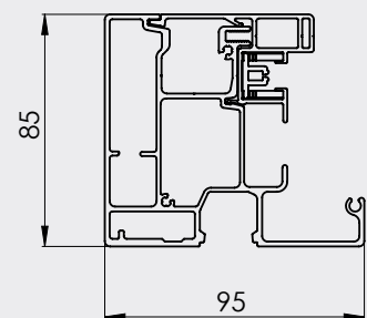
Sidoskena
