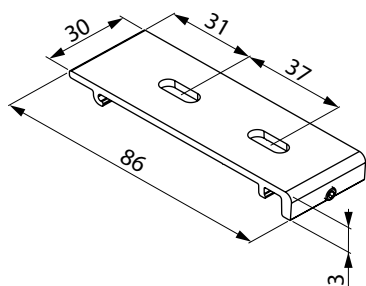
Konsol Montageskena
