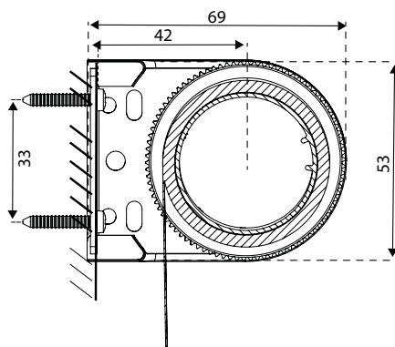
Väggmontage - LR-reglage
