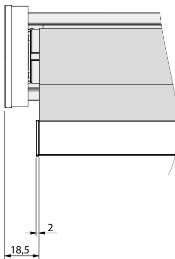
Mjukstängande/Motor
