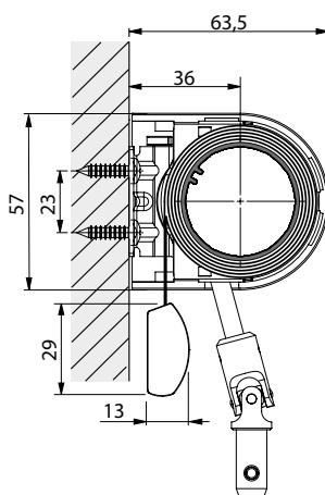
Väggmontage - Vevreglage
