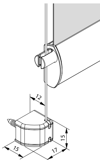
Väggmonterad
