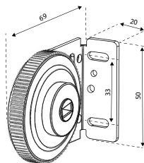
Montagekonsol LR-reglage
