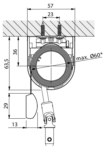
Takmontage - Vevreglage
