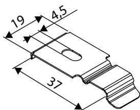
Clips för kassett och mörkläggande skena
