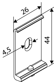
Konsol montageskena - Vevreglage
