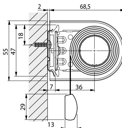
Väggmontage - Mjukstängande
