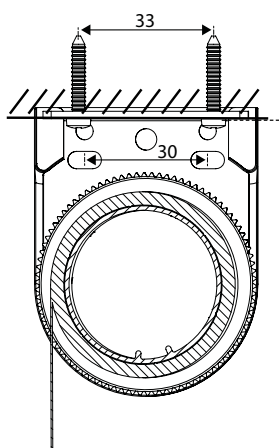
Takmontage - LR-reglage
