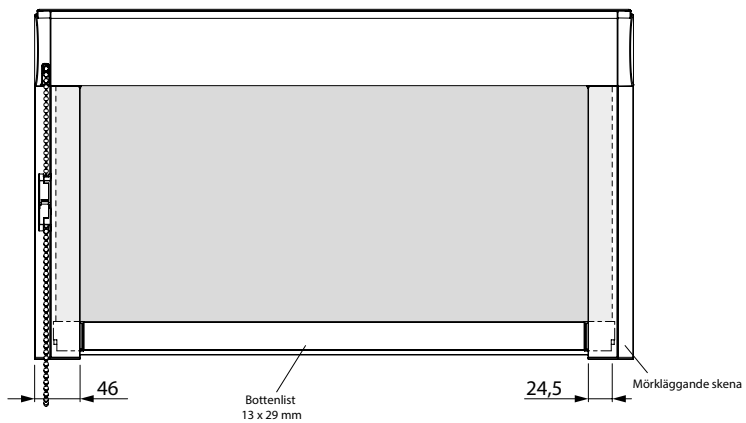
Kulkedja
