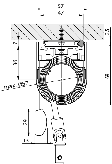
Takmontage - Vevreglage
