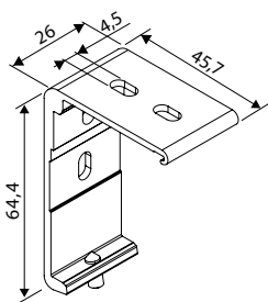
Konsol kassett - Vevreglage
