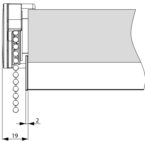
Kulkedja
