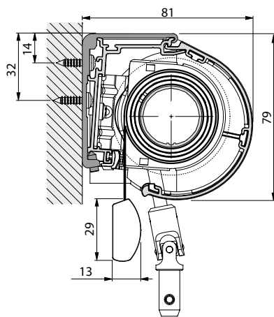
Väggmontage - Vevreglage
