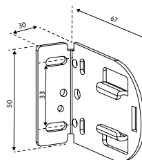
Montagekonsol LR-reglage
