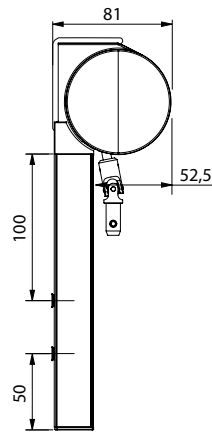
Clipsmontage - Vevreglage
