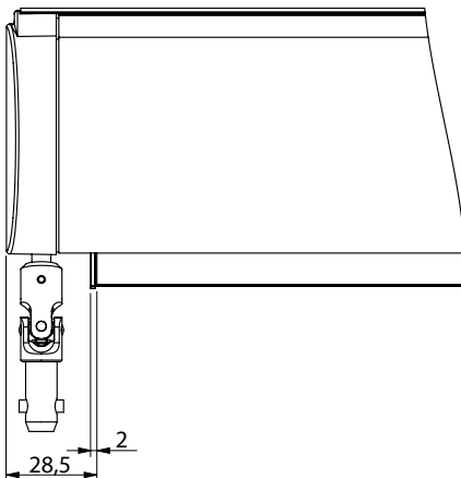
Vevreglage
