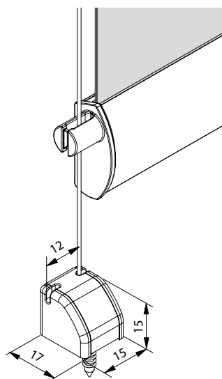
Bottenmonterad
