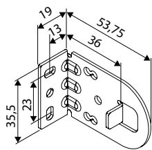
Konsol 36 (standard)
