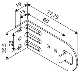
Konsol 60
