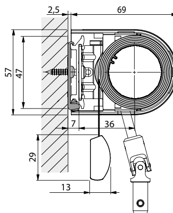
Väggmontage - Vevreglage
