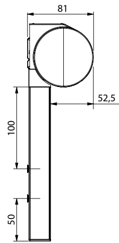
Clipsmontage - Motor
